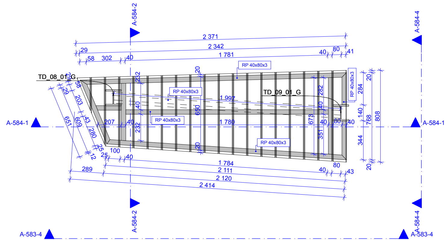
A-584 Rzut ławki 1:20
